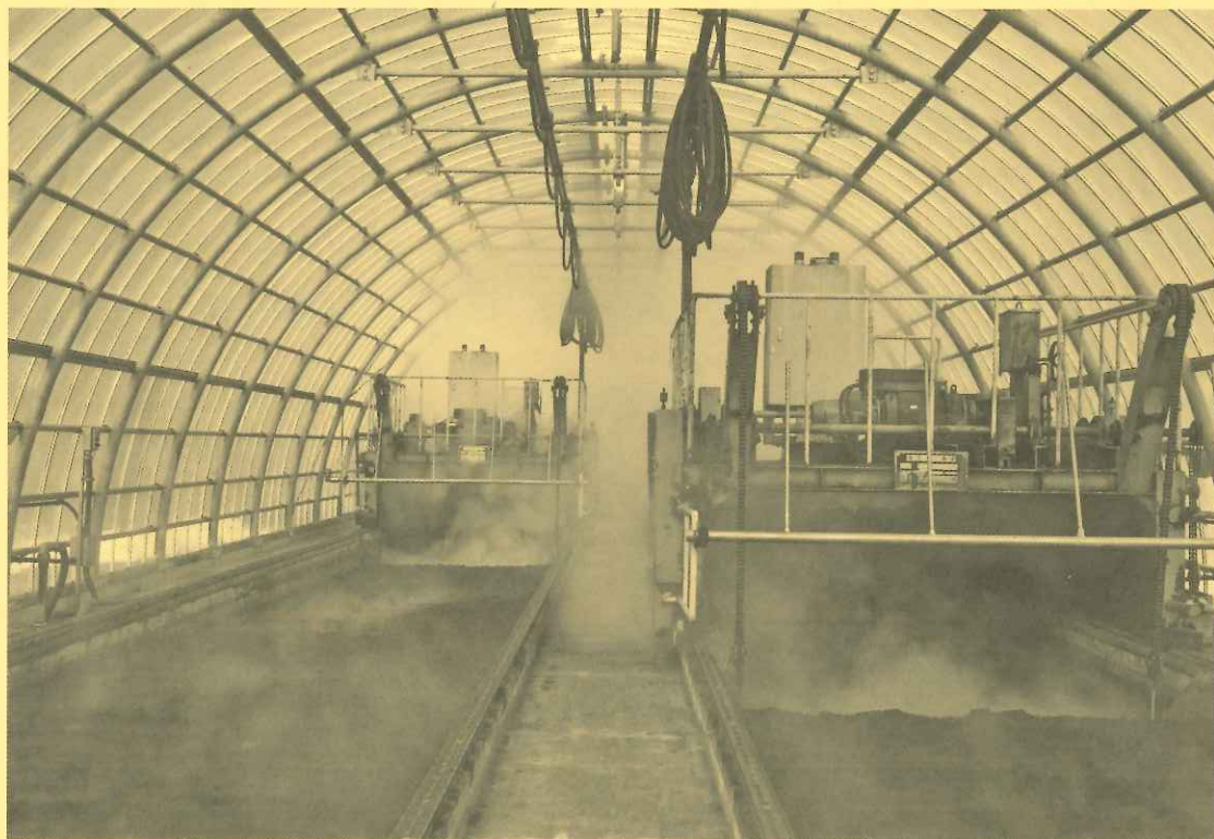
チェーンスクープ型攪拌機による攪拌
