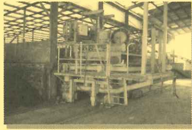
2次発酵槽：機械攪拌発酵1週間
